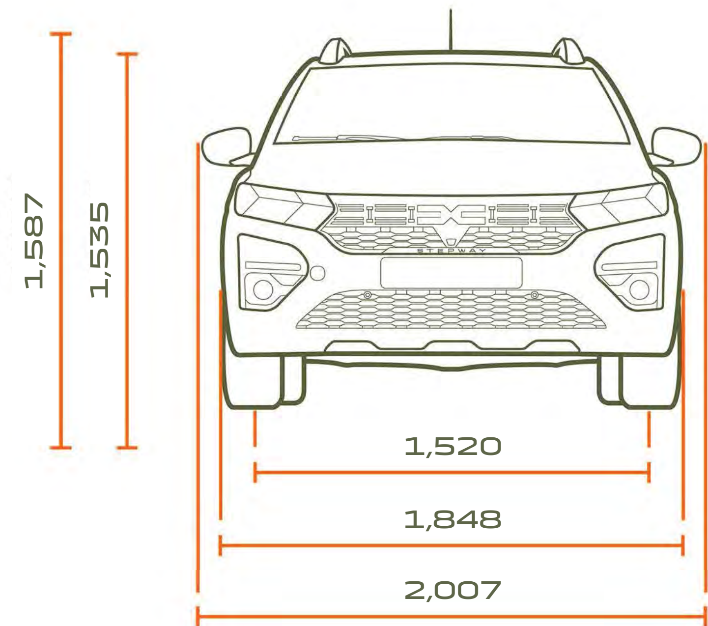
מבט קדמי
