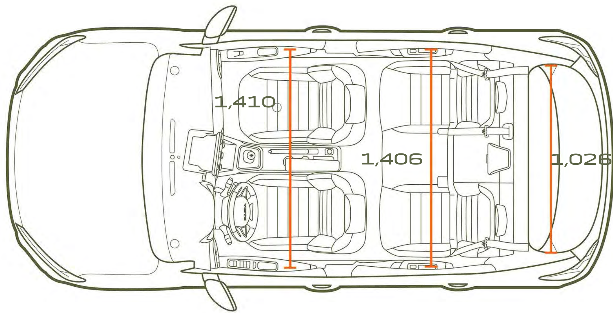
מבט על
