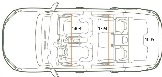
מבט עילי
