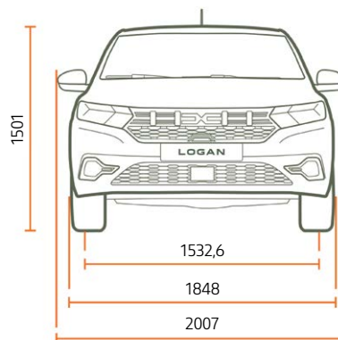
מבט מלפנים
